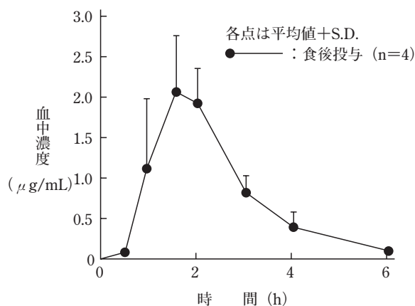
100mg単回経口投与時のアクタリットの血中濃度推移
